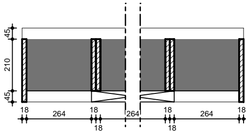
VUE EN COUPE CC
