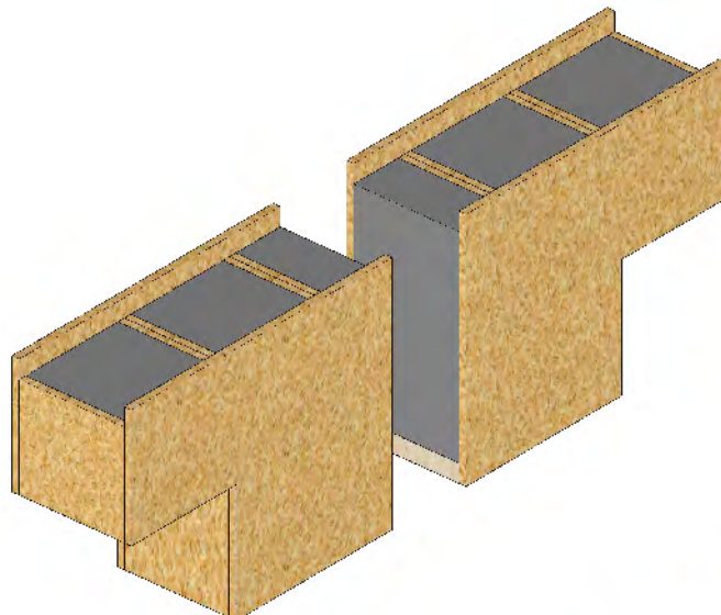
VUE EN PERSPECTIVE
